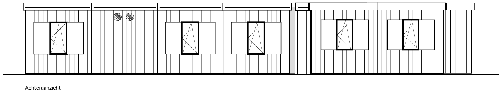
Gevelaanzichten Gebouw Scouting - Oss (versie 3)
