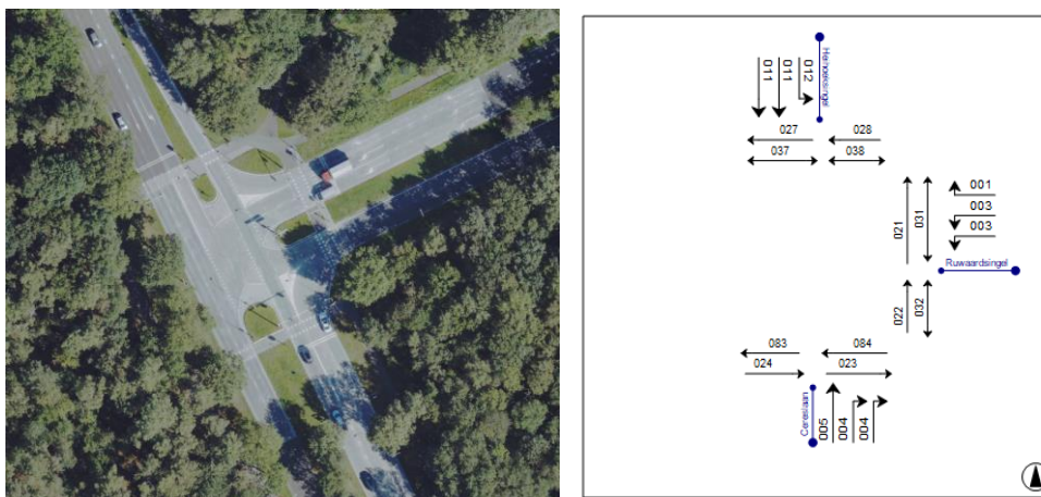
Figuur 3.5: Luchtfoto Heihoeksingel – Ruwaardsingel – Cereslaan en schematische signaalgroepindeling
